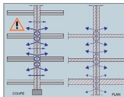
En raison de leur épaisseur, les parois creuses sans ancrage peuvent être à l'origine d'une importante diffusion latérale du bruit, tant verticalement (coupe) qu'horizontalement (plan).
